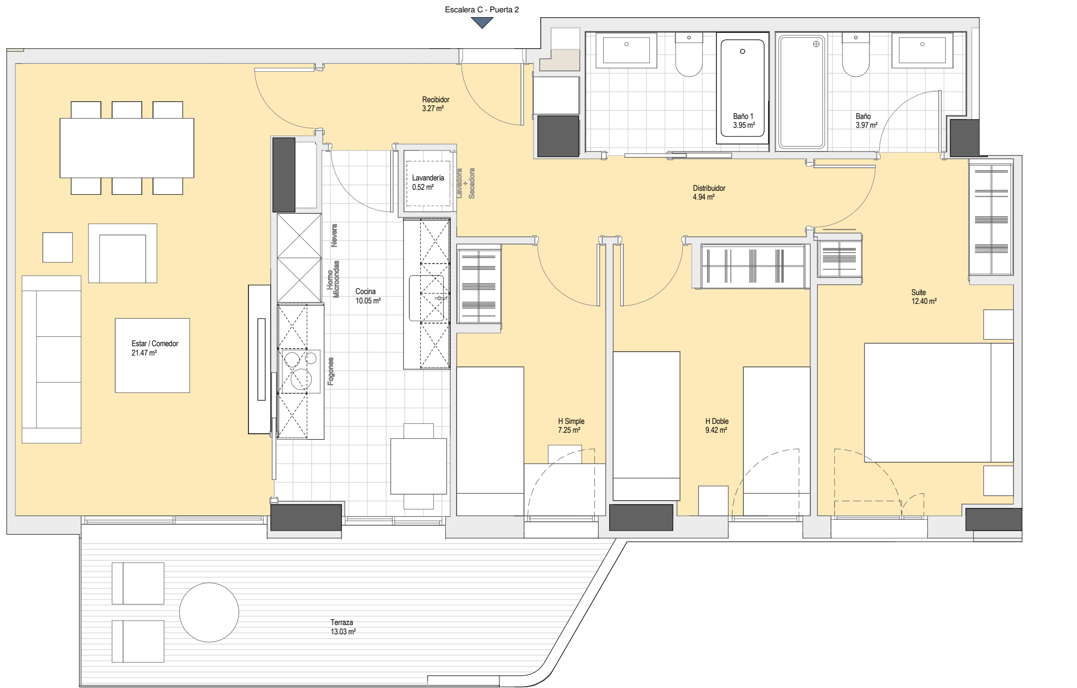
Vivienda Tipo 3D04 1:50 (A3)
