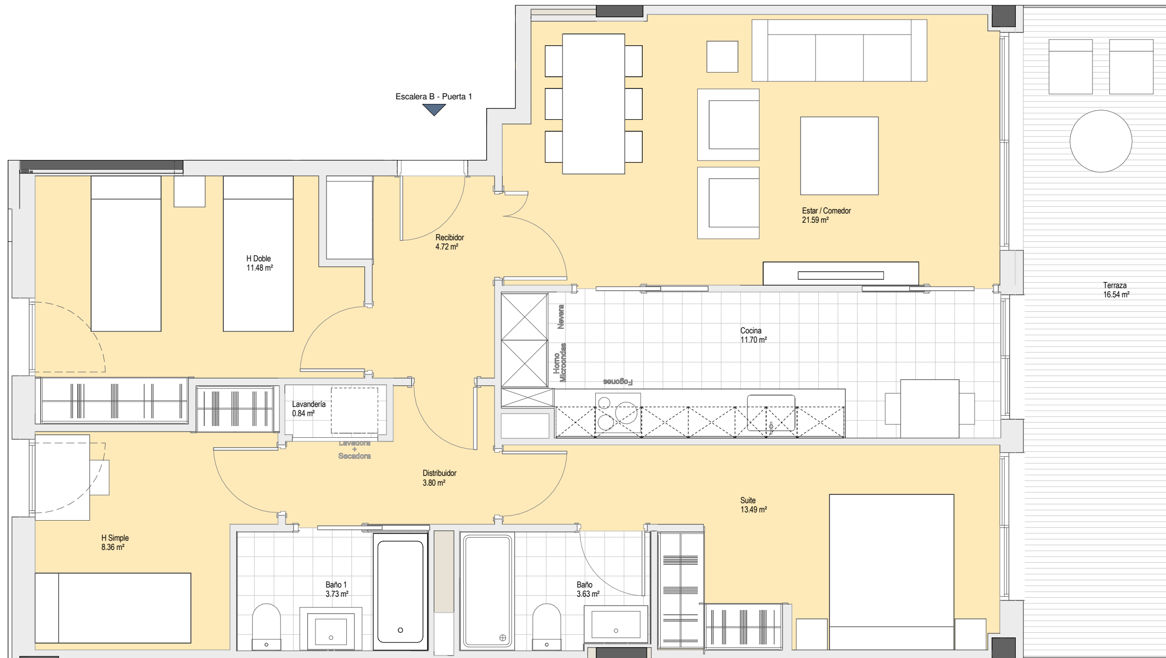
Vivienda Tipo 3D03 1:50 (A3)
