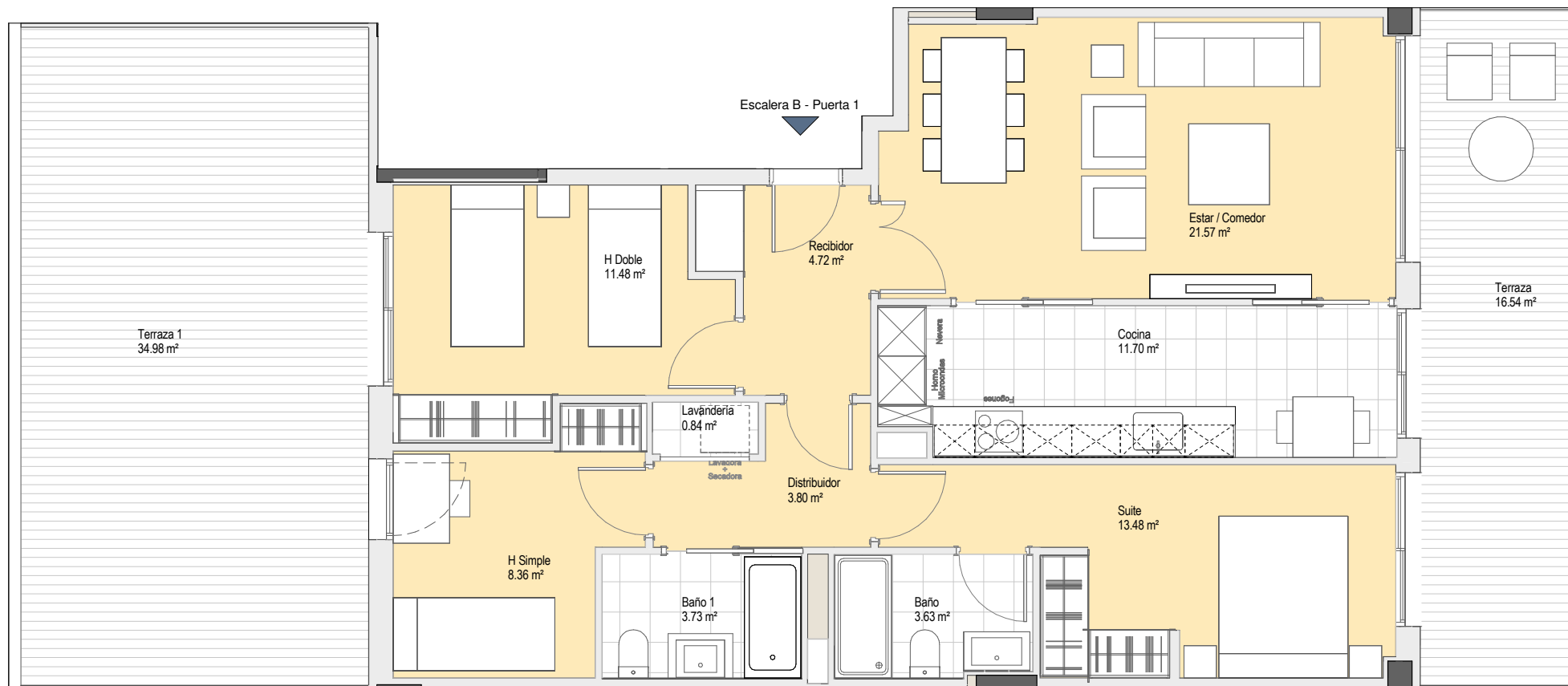
Vivienda Tipo 3D03 1:75 (A3)
