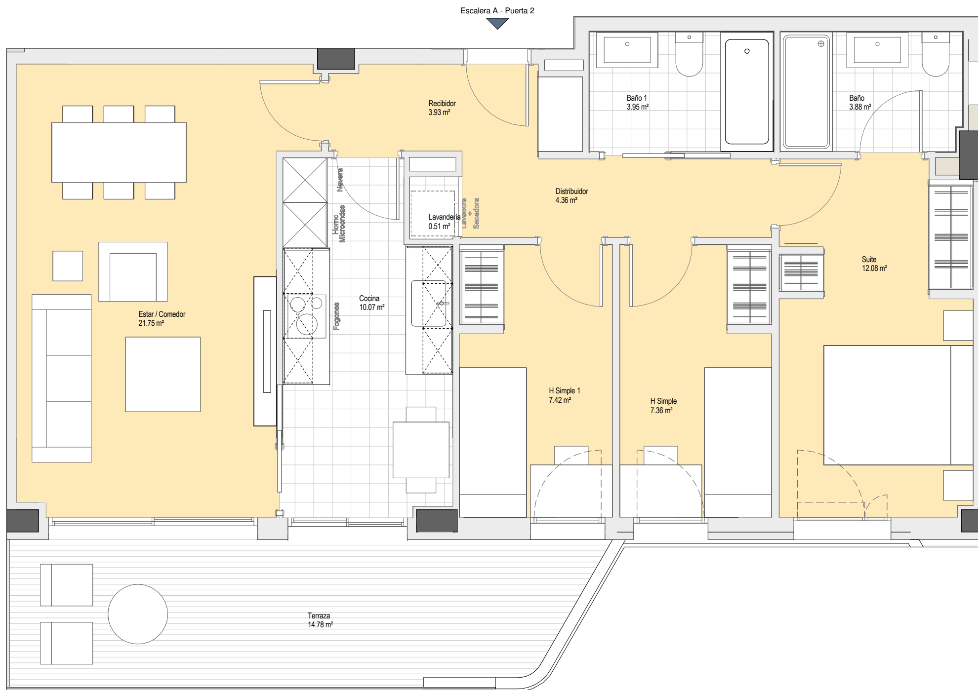
0 1 2 3 5 1:50 (metros)
