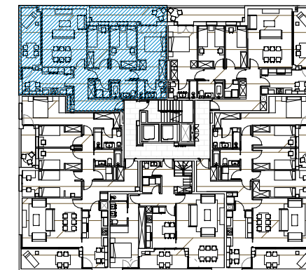
PLANTA PRIMERA
